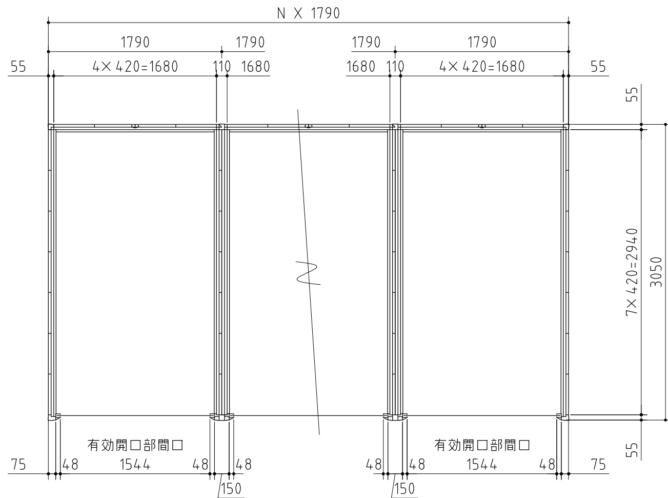
平面図
