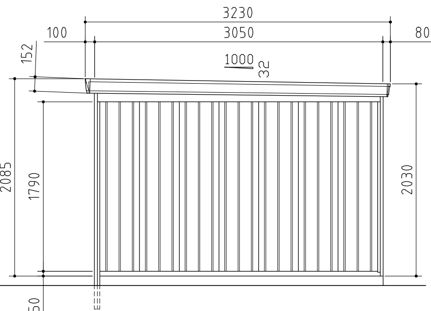
側面図
